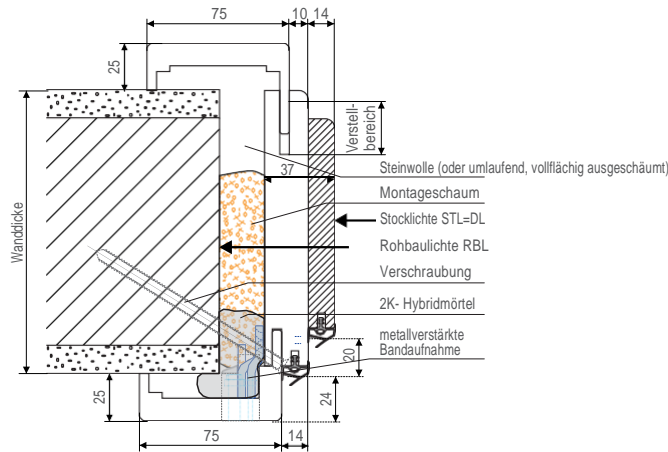
Schnitt G1 - G2
